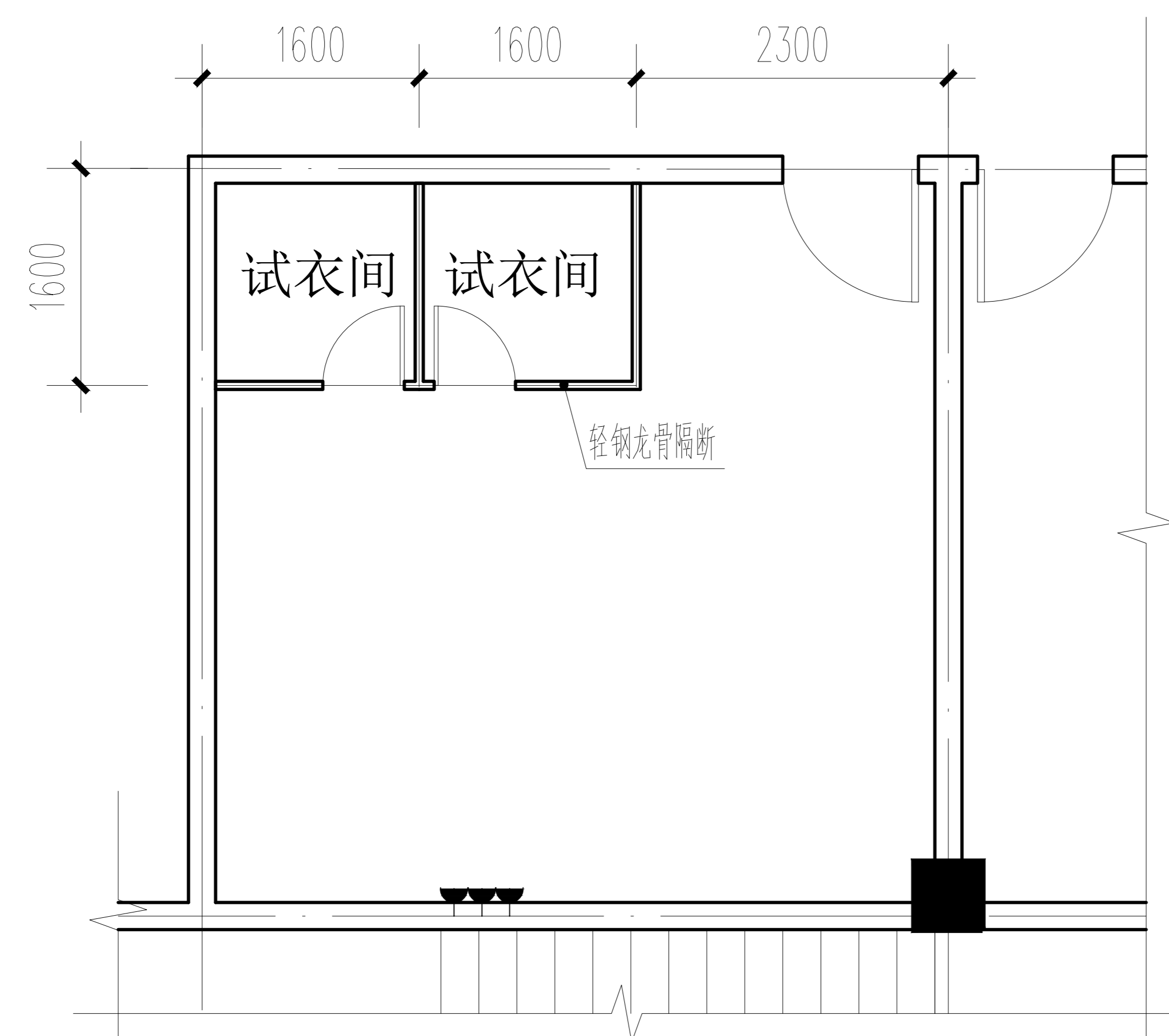
直播办公室 1:100 37.16m 2
