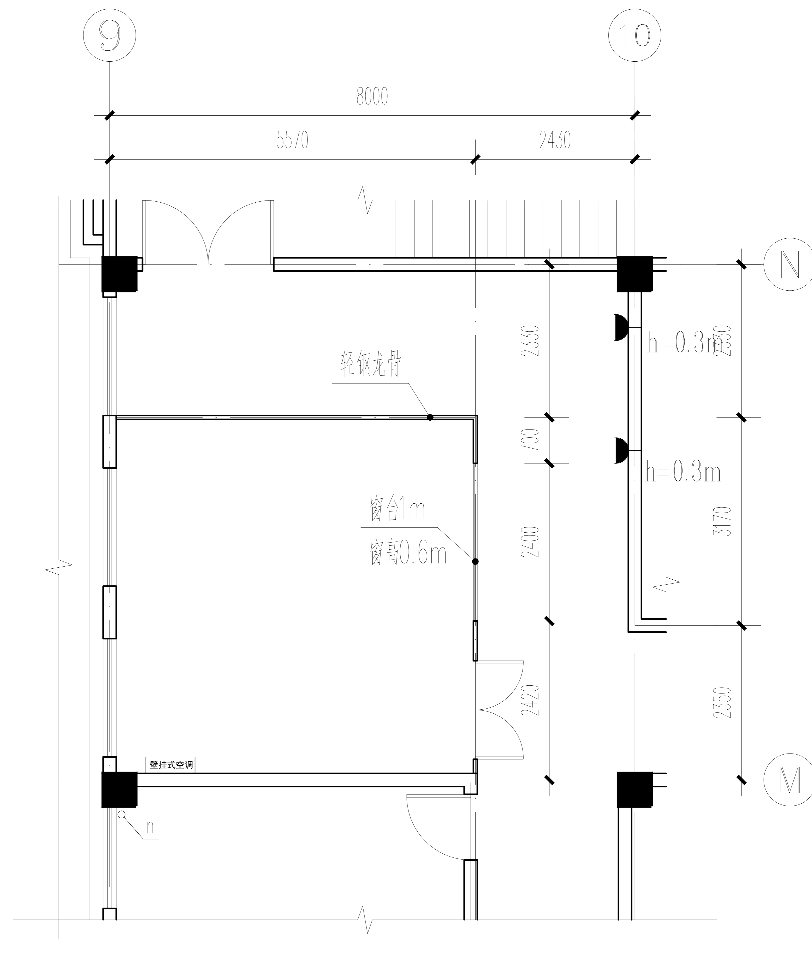
直播会议办公室 1:100 29.32m 2
