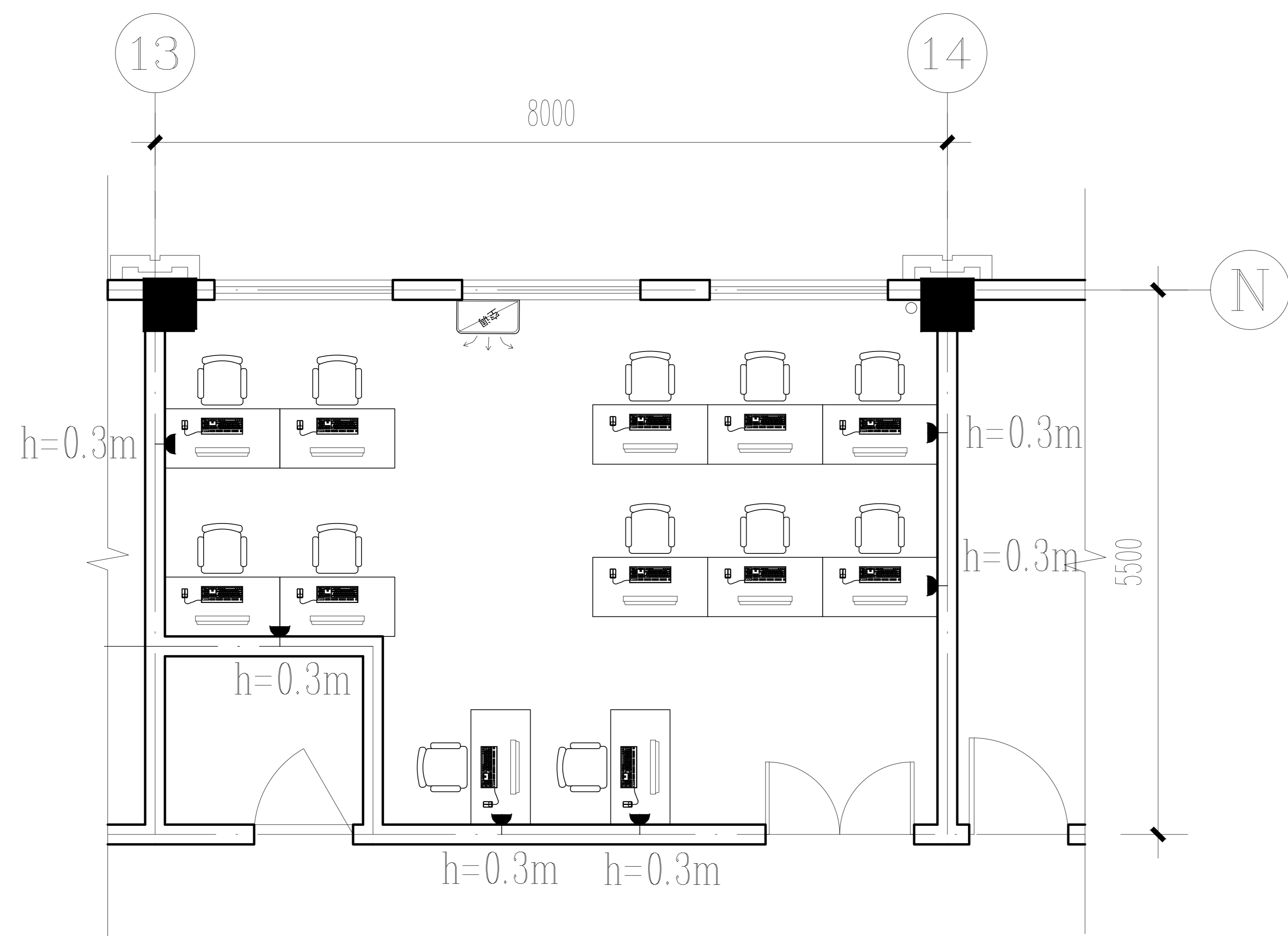
直播办公室 1:100 37.16m 2
